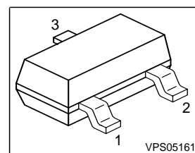
SOT-23
